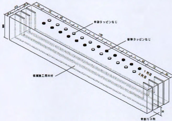
図1.1 木材の外観とタッピンねじの配置 (単位：mm)
