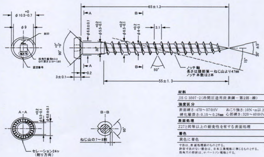
図1.2 タッピンねじSTS・C65 (単位：mm)
